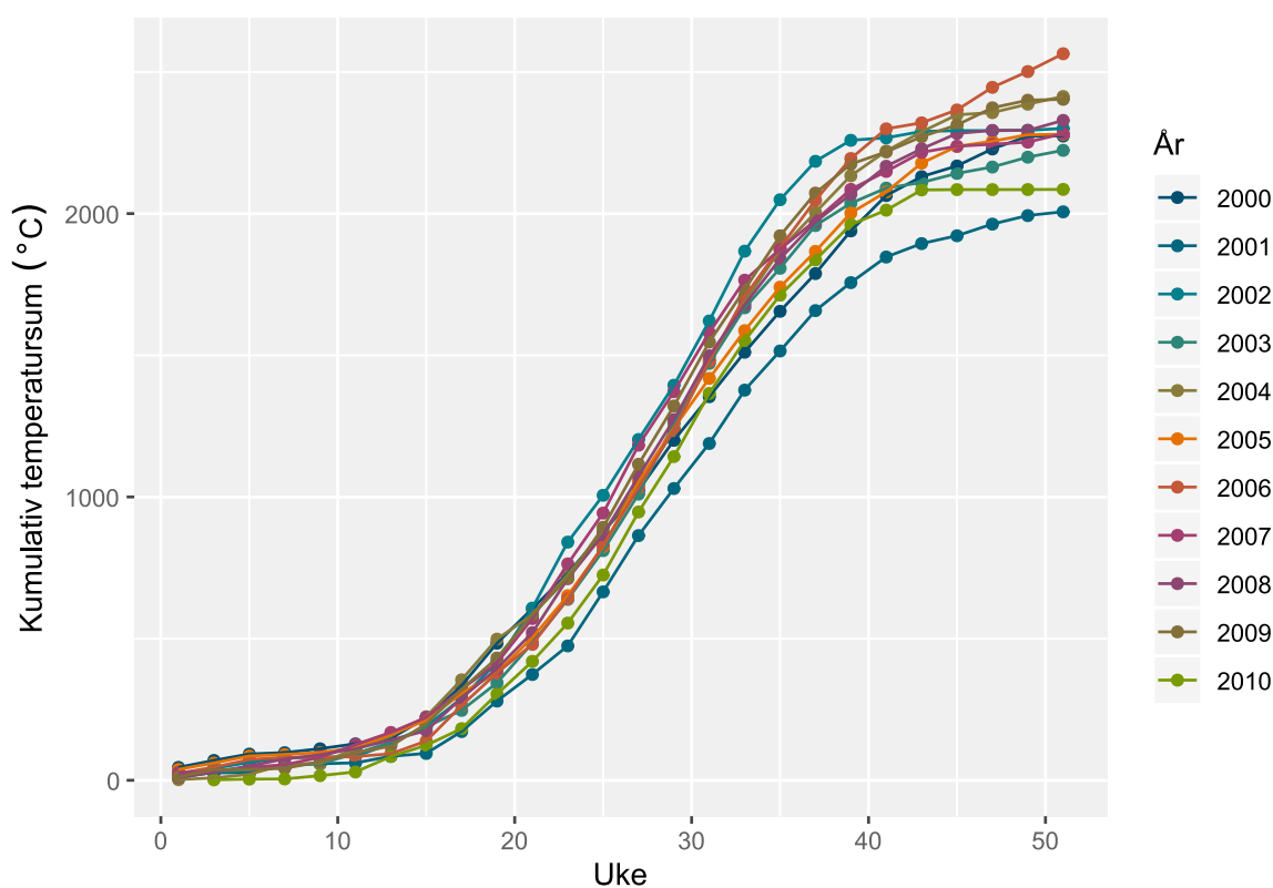
Figur 26. Kumulativ daglig temperatur for dager med middeltemperaturer over null, for hver to-ukersperiode mellom år 2000 og 2010 i Lokalitet A «Fjølstad».
