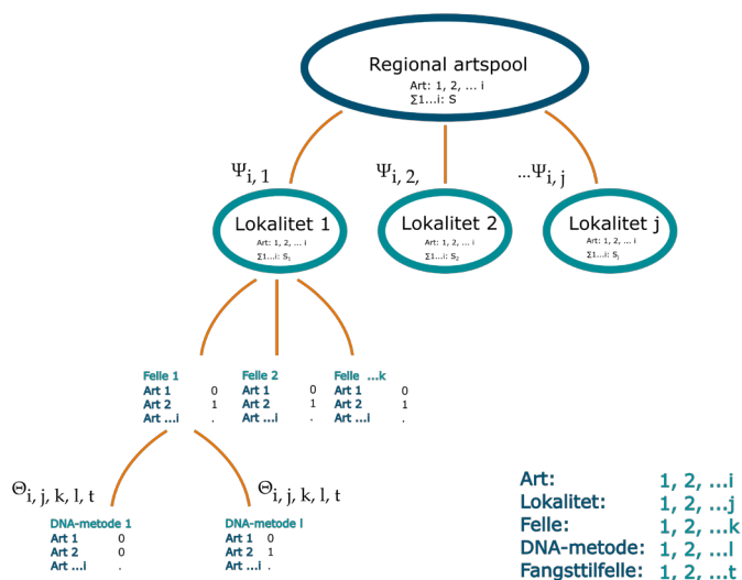
Figur 7. Skjematisk illustrasjon over forekomst-deteksjonsmodellen som ble brukt. Den regionale artspoolen har et totalt artsantall S , som blir estimert fra modellen. Hver art ( i ) forekommer på en gitt lokalitet ( j ) ved et samplingstilfelle ( t ) med en art og lokalitetsspesifikk forekomstsannsynlighet \Psi_{ij} . Hver felle ( k ) samler fra den lokale forekomsten og insektene identifiseres med metodikk I. Metodikken oppdager de artene som er tilstede i hver lokalitet med sannsynlighet \Theta_{ijklt} .
