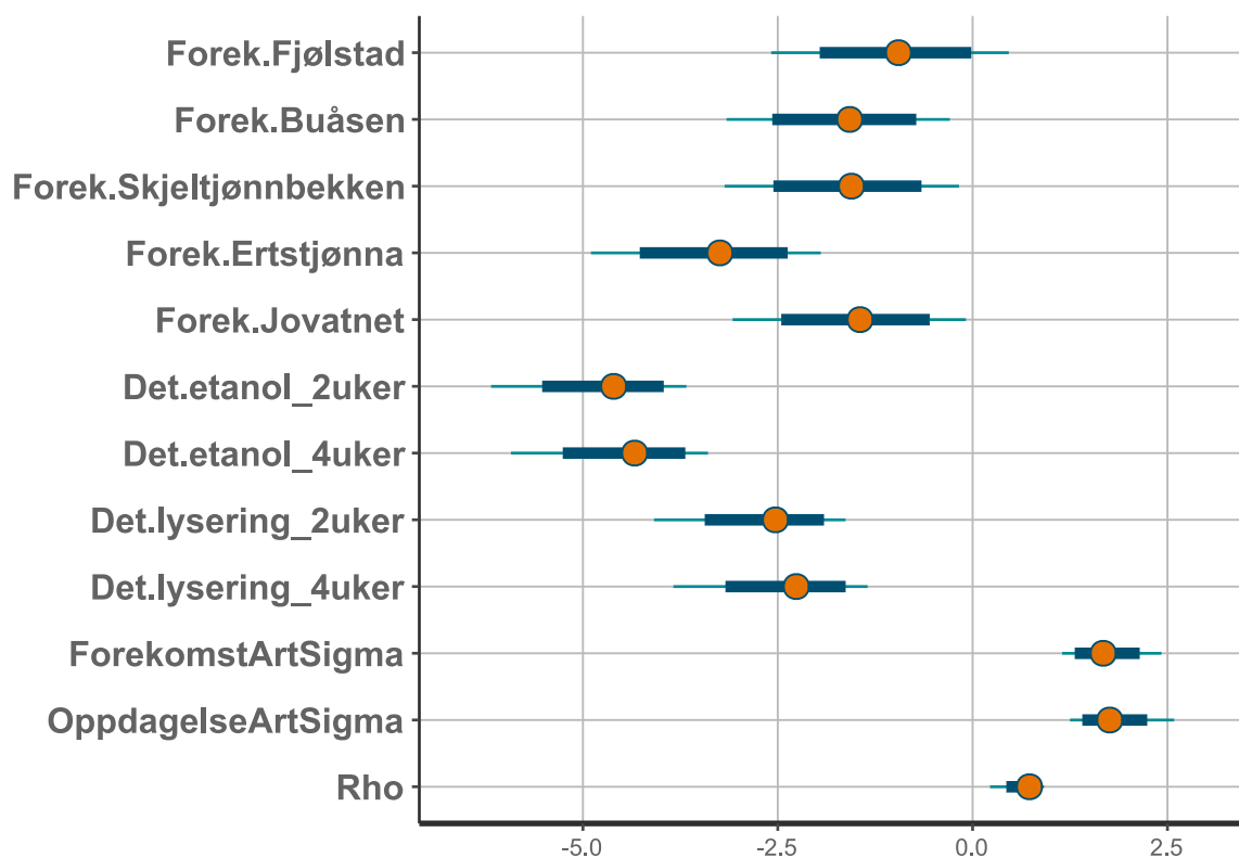
Figur 18. Parameterestimat for occupancy-detection modellen av blomsterfluer (Syrphidae). Verdiene vises i logit-skala. Forek.Lokalitet angir den gjennomsnittlige forekomstsannsynligheten for en blomsterflue i hver enkelt lokalitet. Det.etanol_2uker angir deteksjonssannsynligheten for en gjennomsnittlig blomsterflue i filtrert etanol ved to ukers fellefangst. Tilsvarende deteksjonssannsynlighet vises også for 4 ukers innsamling og i lyserte prøver. ForekomstArtSigma og OppdagelseArtSigma viser variasjonen i forekomst og deteksjonssannsynlighet på artsnivå som standardavvik, og Rho angir samvariasjonen mellom disse.
