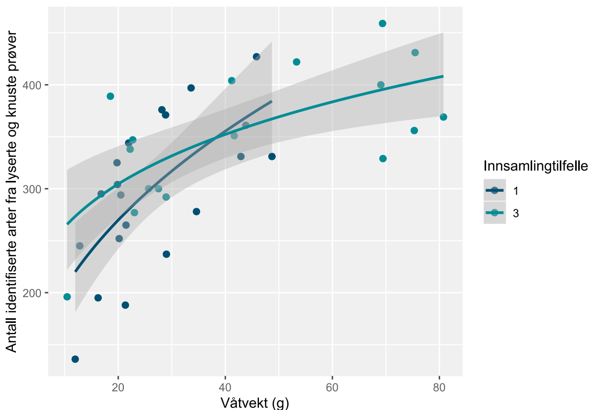
Figur 8. Samsvar mellom total våttvekt i fellefangstene og antall arter identifisert gjennom metastrekkoding av DNA. Linjen representerer modellen \text{Antall arter} \sim \text{intercept} * \text{Våttvekt}^{\text{stigning}} , identifisert gjennom linjer regresjon av \log(\text{arter}) \sim \log(\text{intercept}) + \text{stigning} * \log(\text{våttvekt}) .
