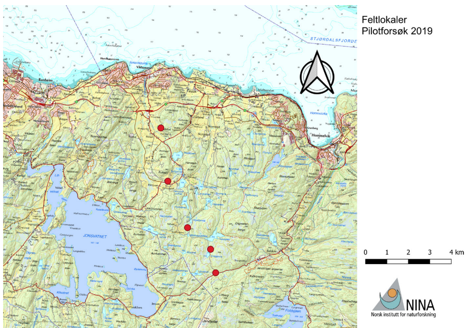
Figur 1. Plassering av prøvelokaliteter for pilotforsøket i 2019. Lokalitetene benevnes A-E fra nord til sydlig retning, der A: Fjølstad, B: Buåsen, C: Skjeltsjønnbekken, D: Ertstjønnna, og E: Jovatnet.
